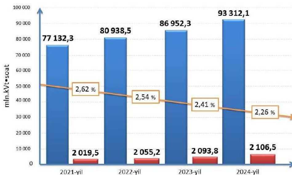
Рисунка 1: Динамика технологических потерь при передаче электроэнергии через магистральные электрические сети в 2021–2024 годах.
